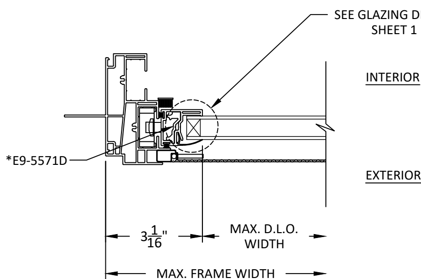
D 6 HORIZONTAL SECTION LEFT JAMB - TOP VENT
