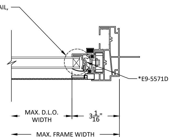
F 6 HORIZONTAL SECTION RIGHT JAMB - TOP VENT
